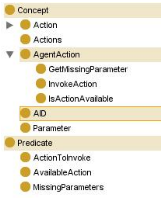
Abbildung 5.1: Ontologie
