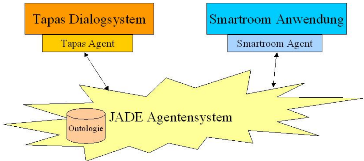
Abbildung 4.1: Übersicht Architektur
